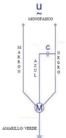
DIAGRAMA DE CONEXIONES
