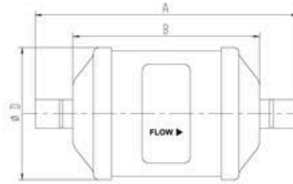
Conexión Soldar
